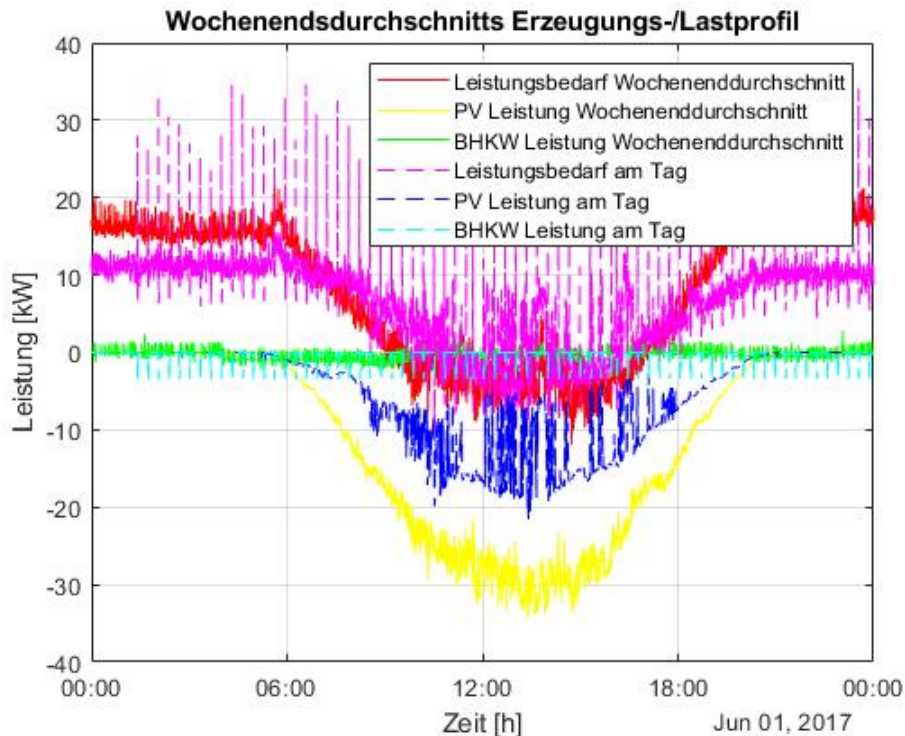
Abbildung 1: Beispiel von Wochenenddurchschnittsprofil (Last/Erzeugung) [eigene Darstellung], siehe [3]
