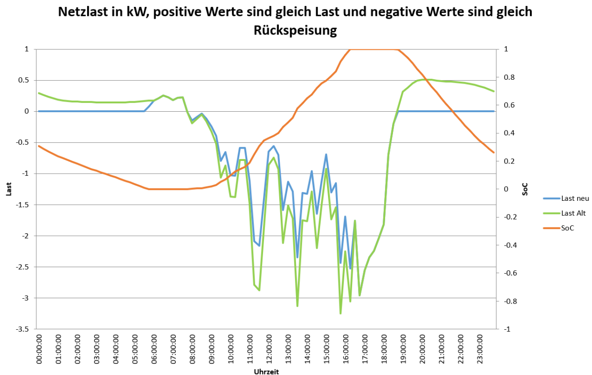
Abbildung 7: Beispiel Szenario: Stufenweise Netzentlastung [3]
