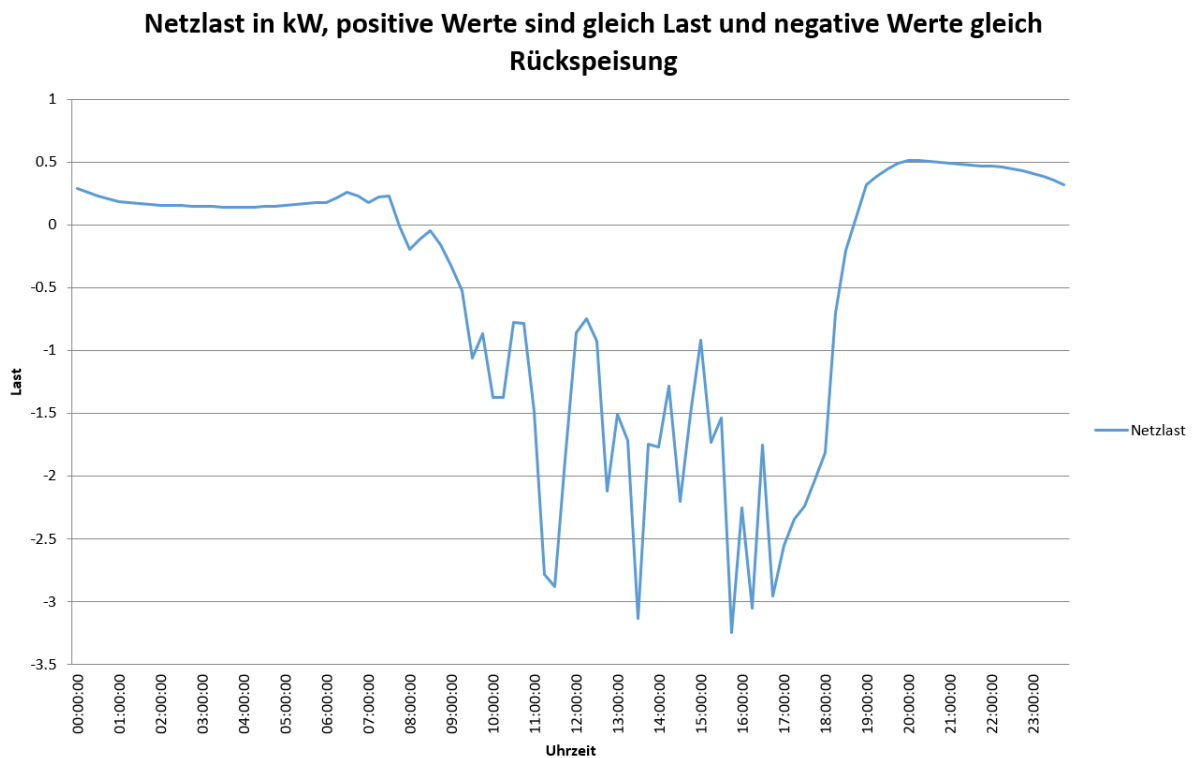
Abbildung 2: Beispiel einer Netzlast über den Tag – Ausgangsdaten [3]
