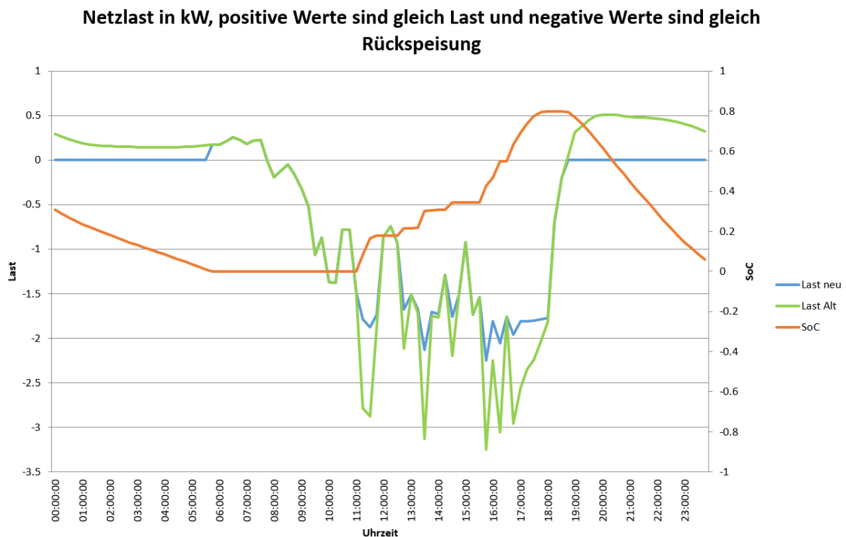
Abbildung 6: Beispiel Szenario: Leistungsbegrenzung [3]
