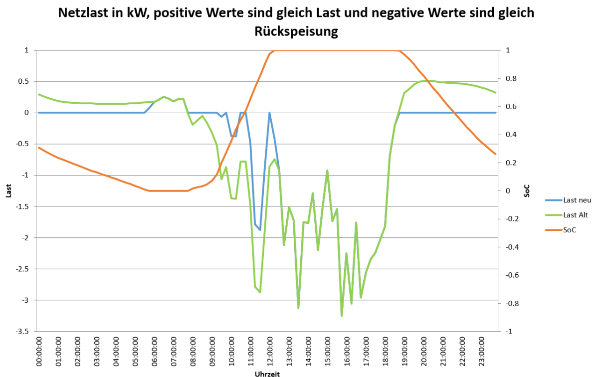
Abbildung 5: Beispiel Szenario: Maximierung des Eigenverbrauchs [3]
